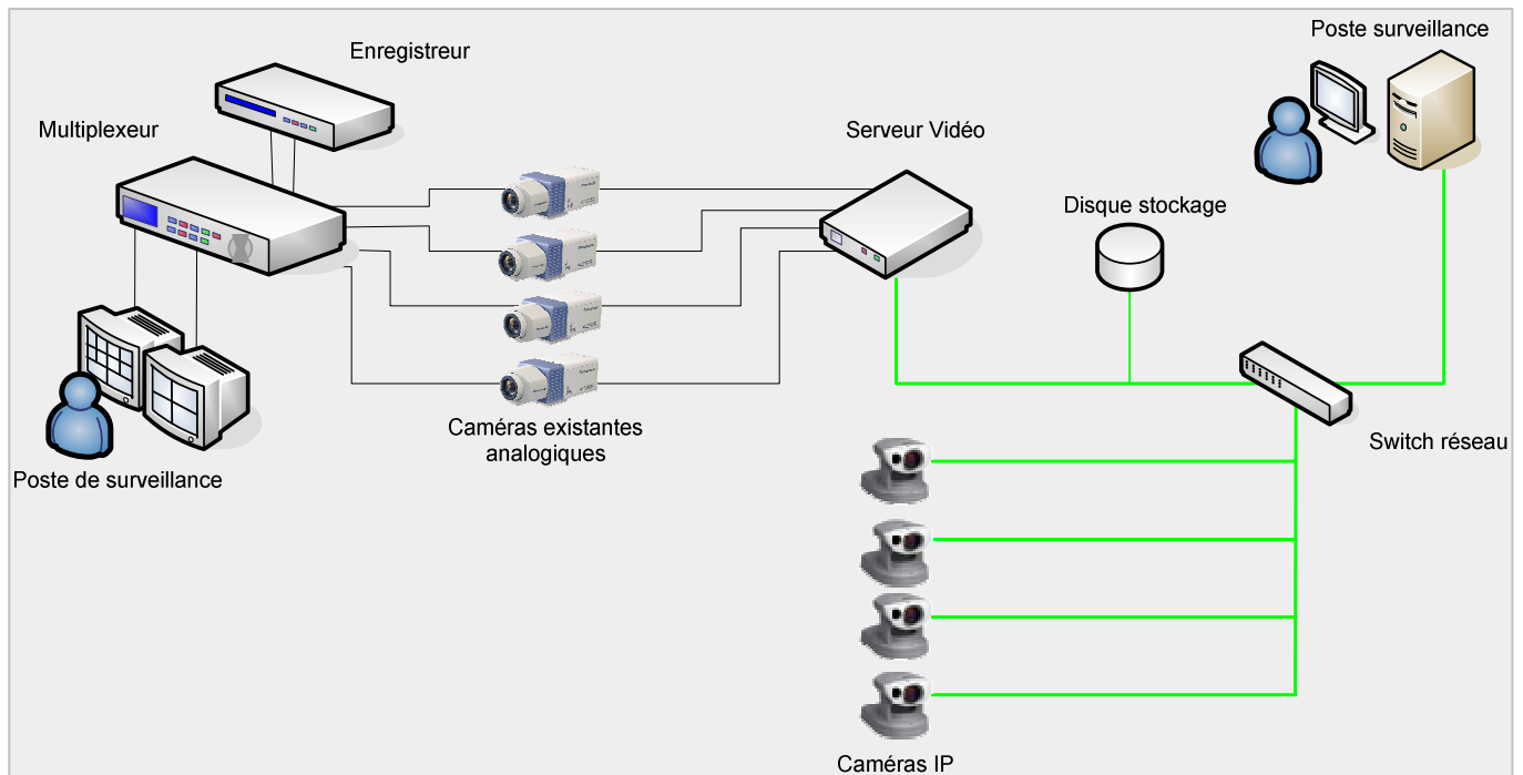
Figure 2 : Intégration d'un système analogique existant avec la technologie IP
